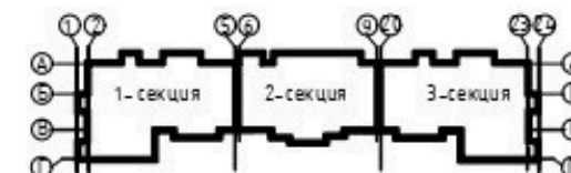
Схема блокировки
